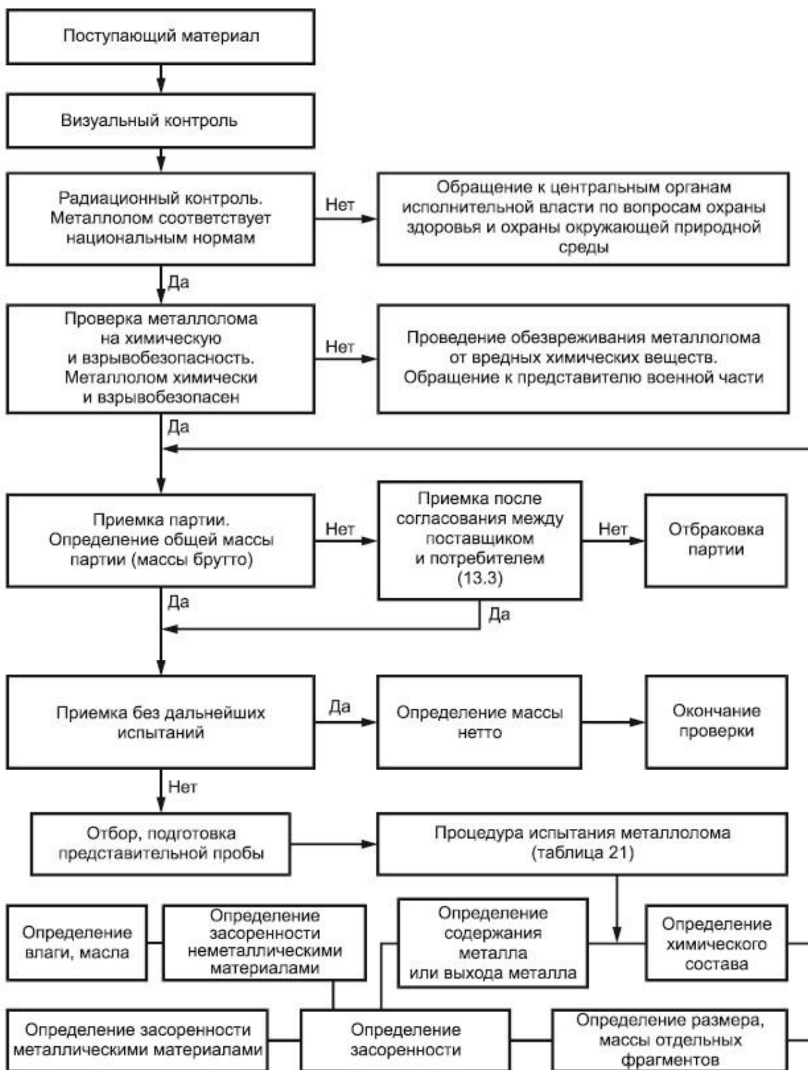
Рисунок 1 - Схема проверки поступающего металлолома
